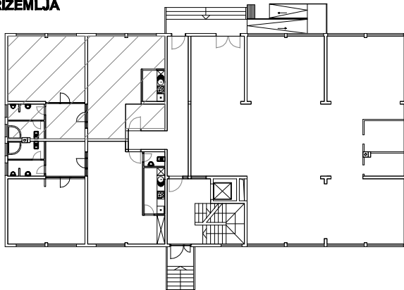
TLOCRT PRIZEMLJA
