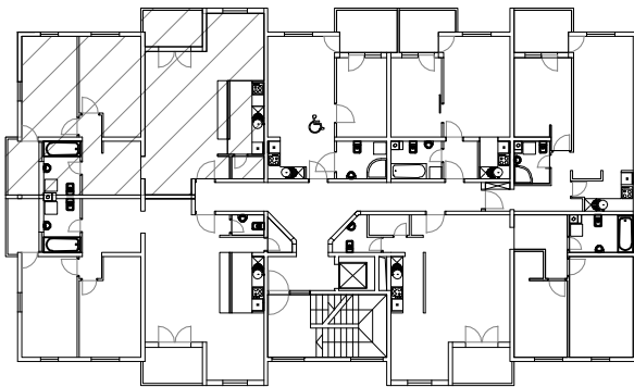
TLOCRT 1. KATA
