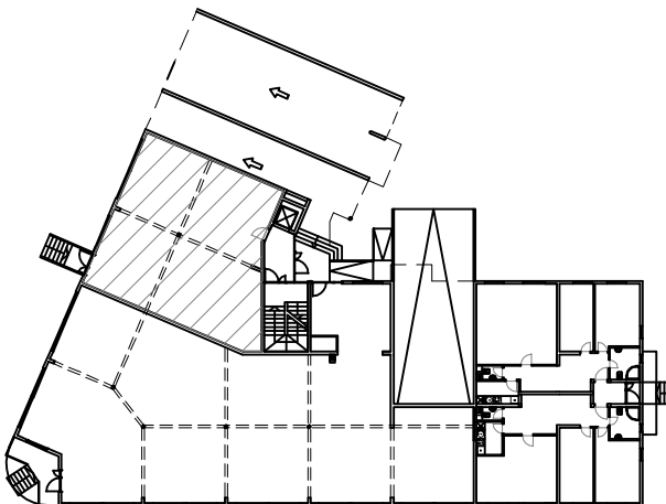
TLOCRT PRIZEMLJA
